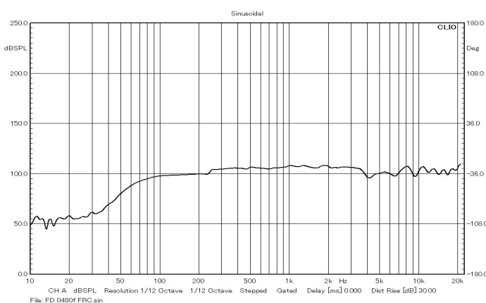
Frequency response curve in Enclosure (* 車両装着時のデータではありません。)
